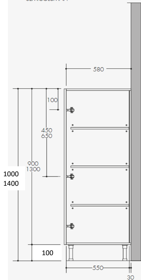
CUERPO SEMICOLUMNA
